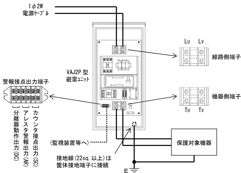
接続図
