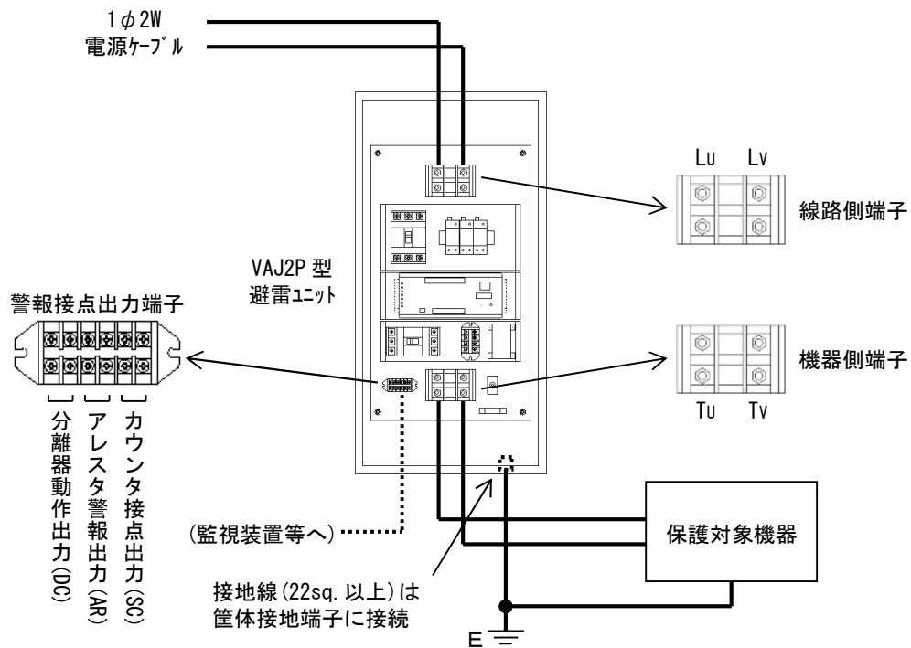
接続図
