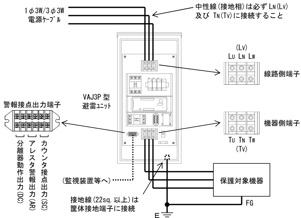
接続図
