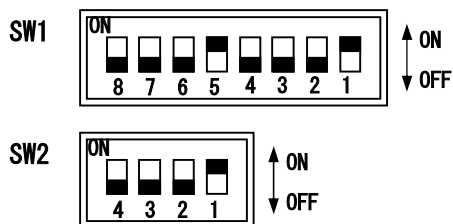
ディップスイッチ設定表
