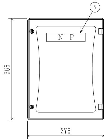
正面図
