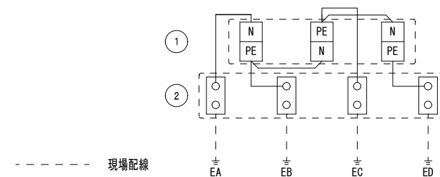
配線参考図
